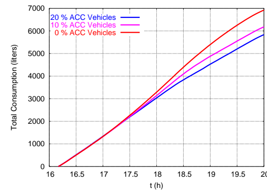
Gesamter Verbrauch auf der simulierten Strecke
