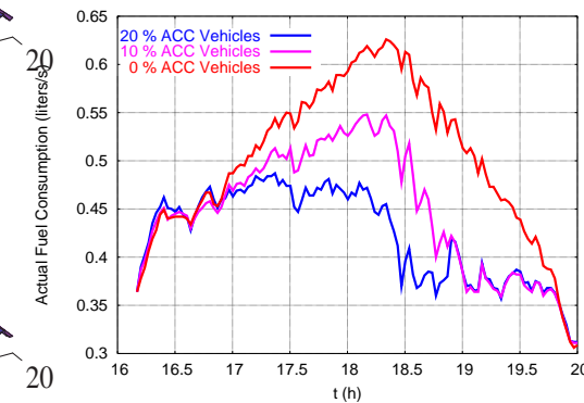
Verbrauchsrate auf der simulierten Strecke
