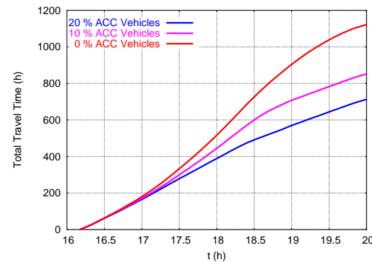
Gesamte Reisezeit auf der simulierten Strecke
