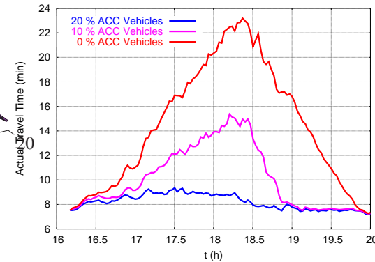
Aktuelle Reisezeit auf der simulierten Strecke
